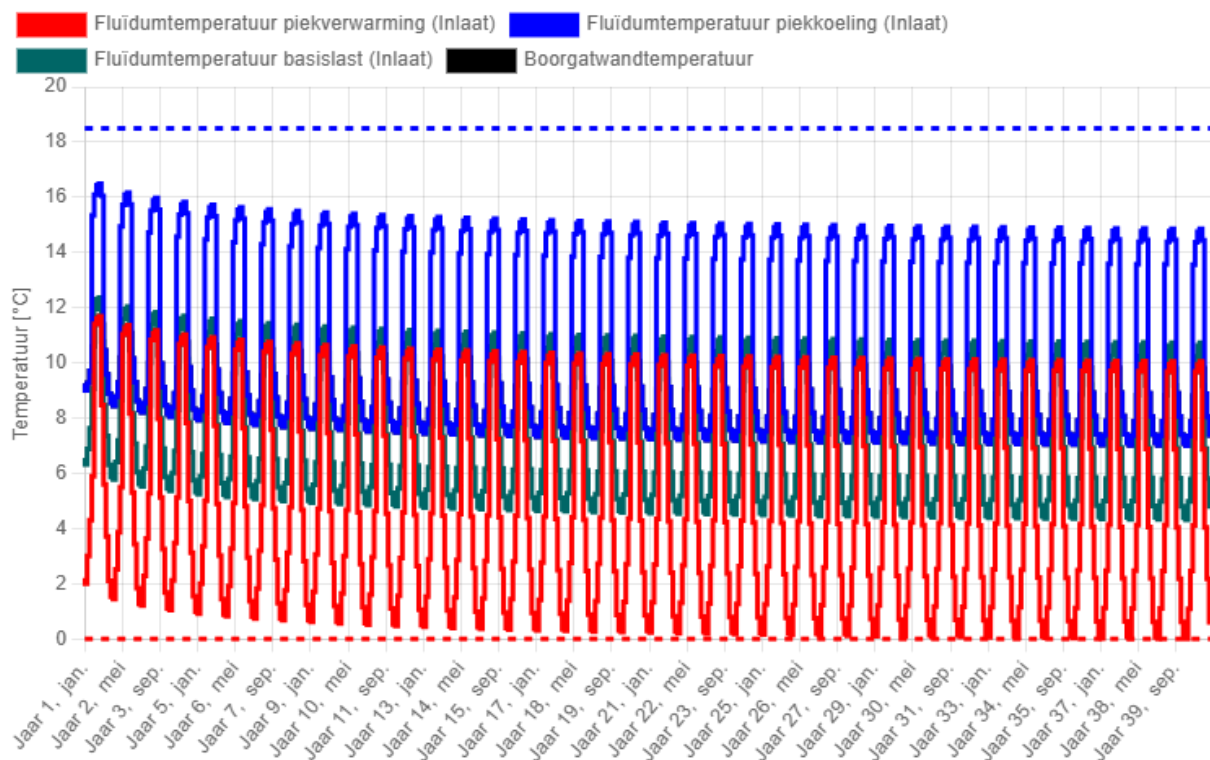
Figuur 2: Voorbeeld van een simulatie met een periode van 40 jaar. De bodem is duidelijk in balans.
